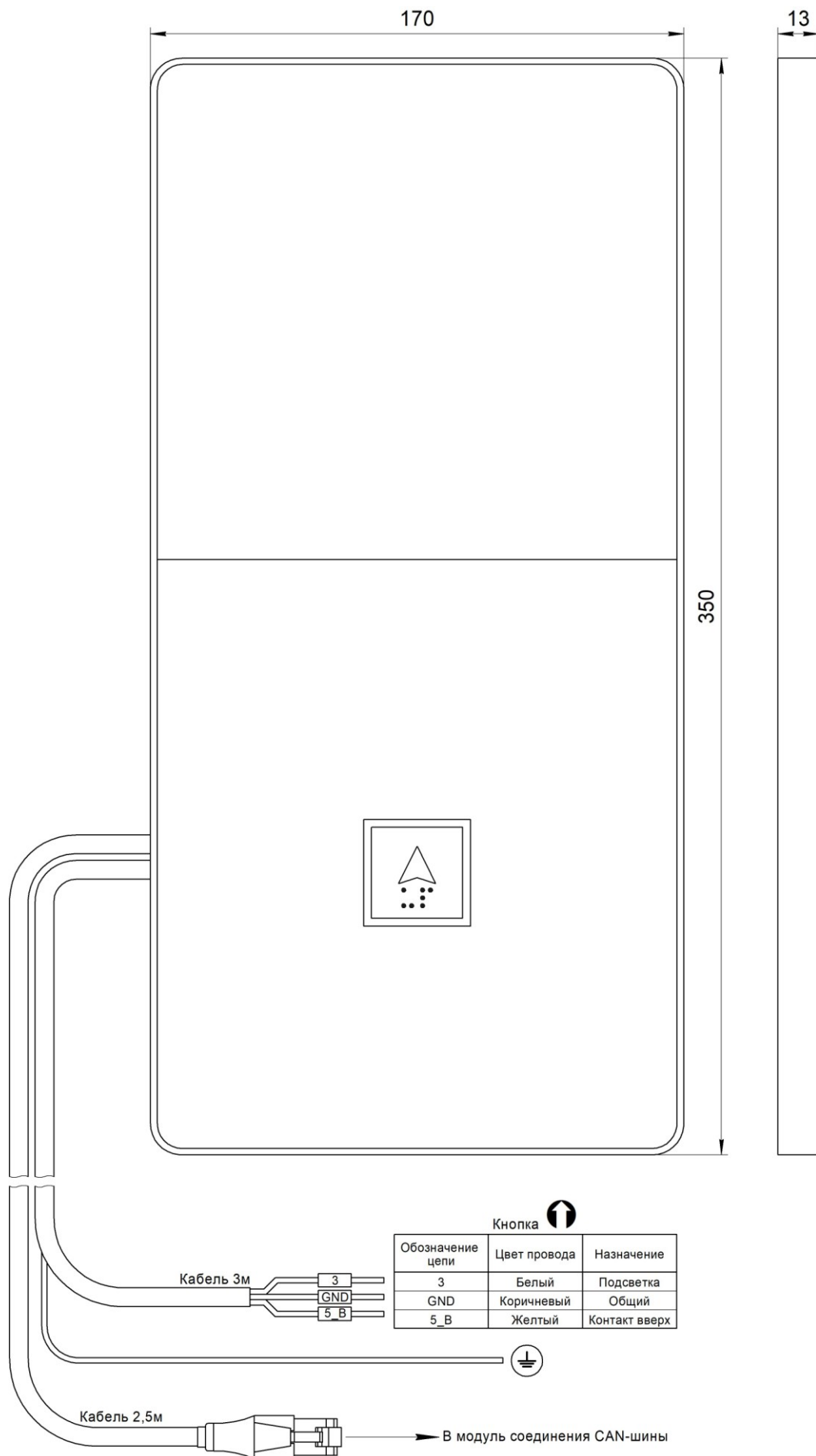
Рис.1 Внешний вид, габаритные и установочные размеры Вызывного поста МАЛАХИТ (жгут RJ45) НШЕК.468381.088
